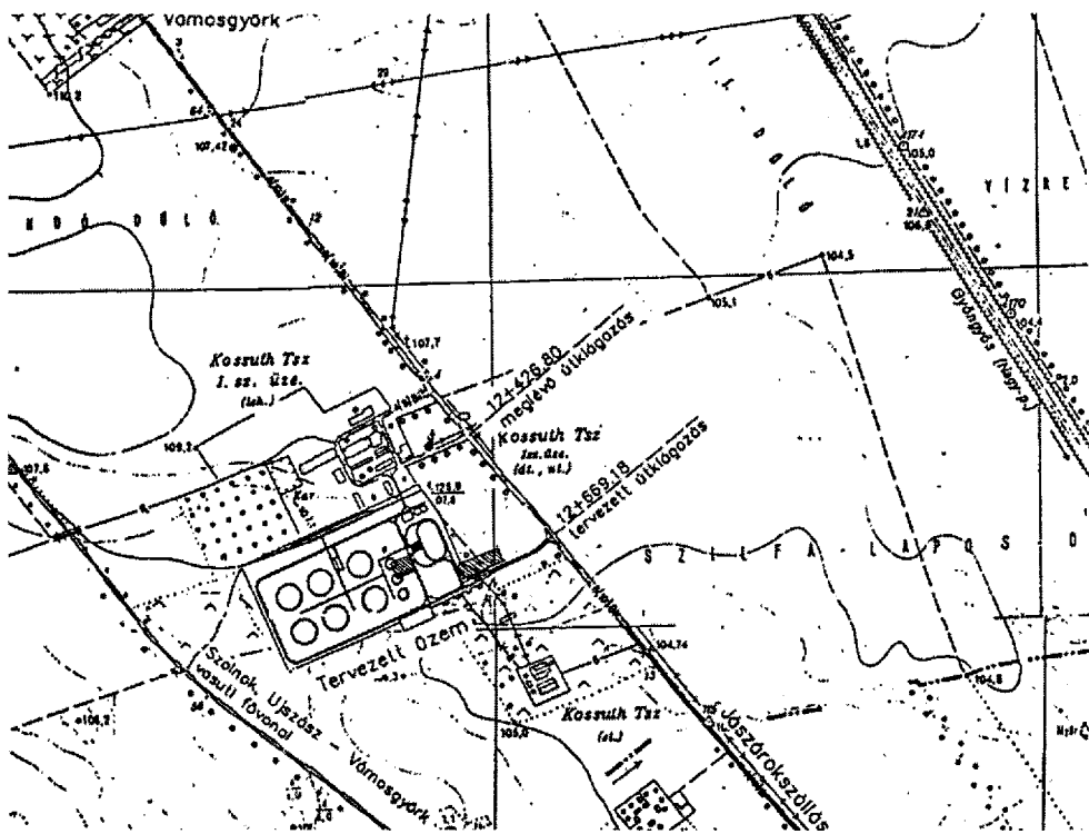
1. kép. 1:10.000 méretarány. A lőhely elhelyezkedése
