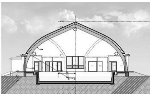
KERESZTMETSZET USZODATÉREN KERESZTÜL
