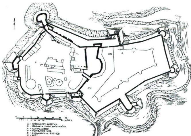
6. ábra PIETRO FERRABOSCO ALAPRAJZA ÉS TERVE 1568-BÓL
