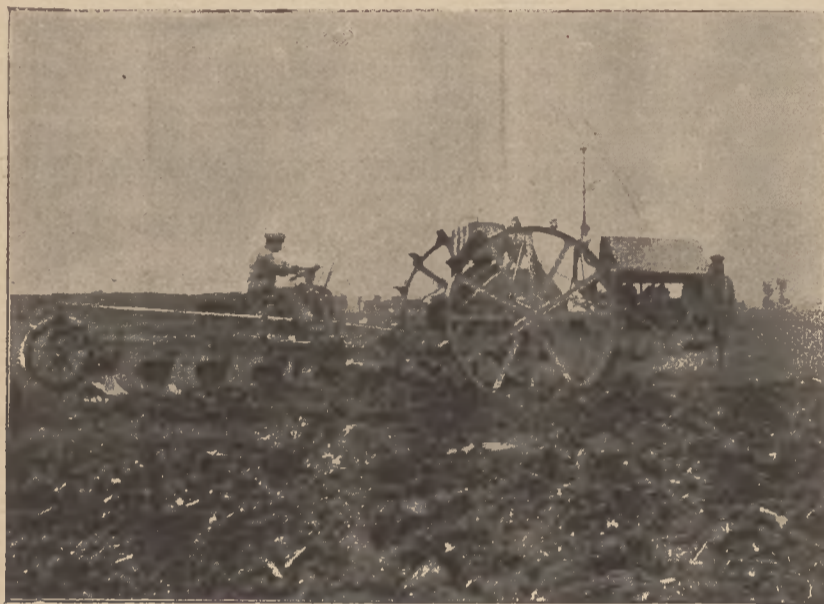
67-ik ábra. Stock benzine motoros eke.
