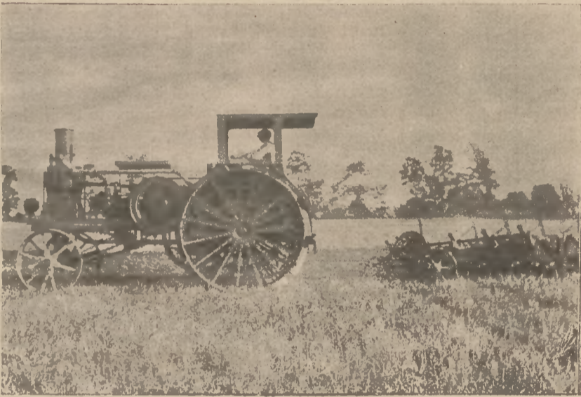
69-ik ábra. Avery benzintraktor.
