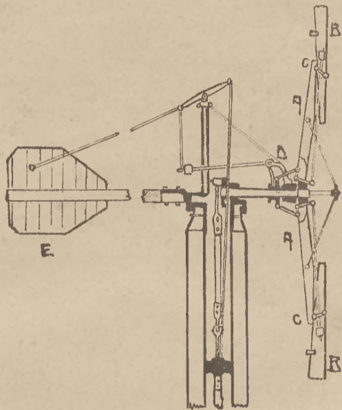
44-ik ábra. „Halady“-féle szélmotor keresztmetszete.
