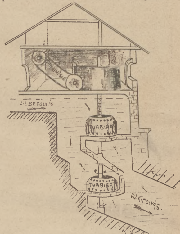
45-ik ábra. Turbinaház két turbinával.
