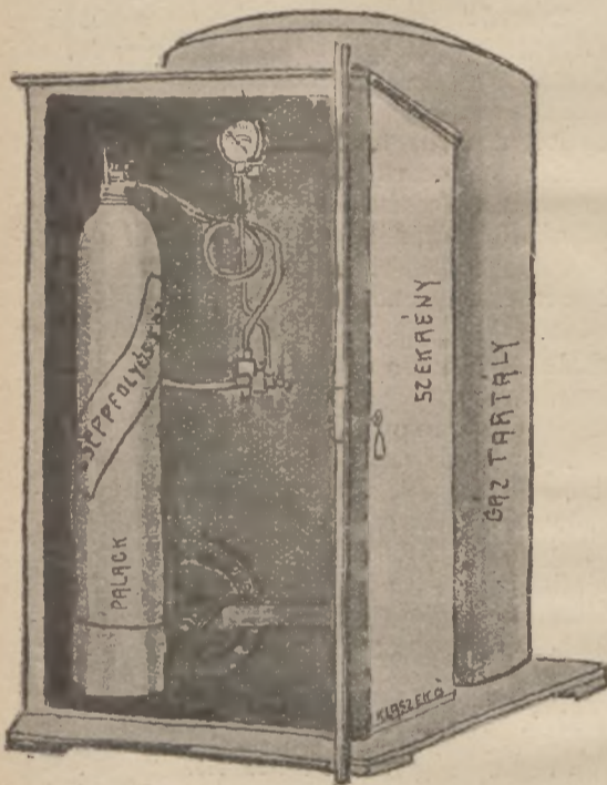
1-ső ábra. Cseppfolyós gáztelep berendezése.
