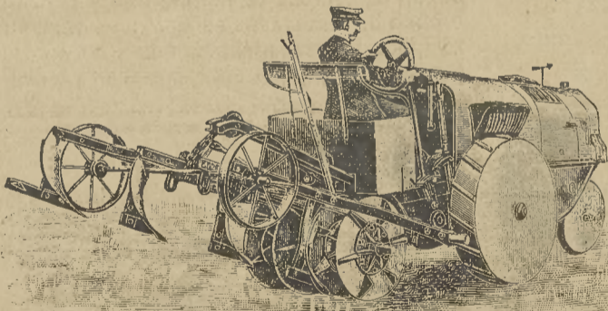
80-ik ábra Pöhl-féle motor mikor csak tárcsáz.
