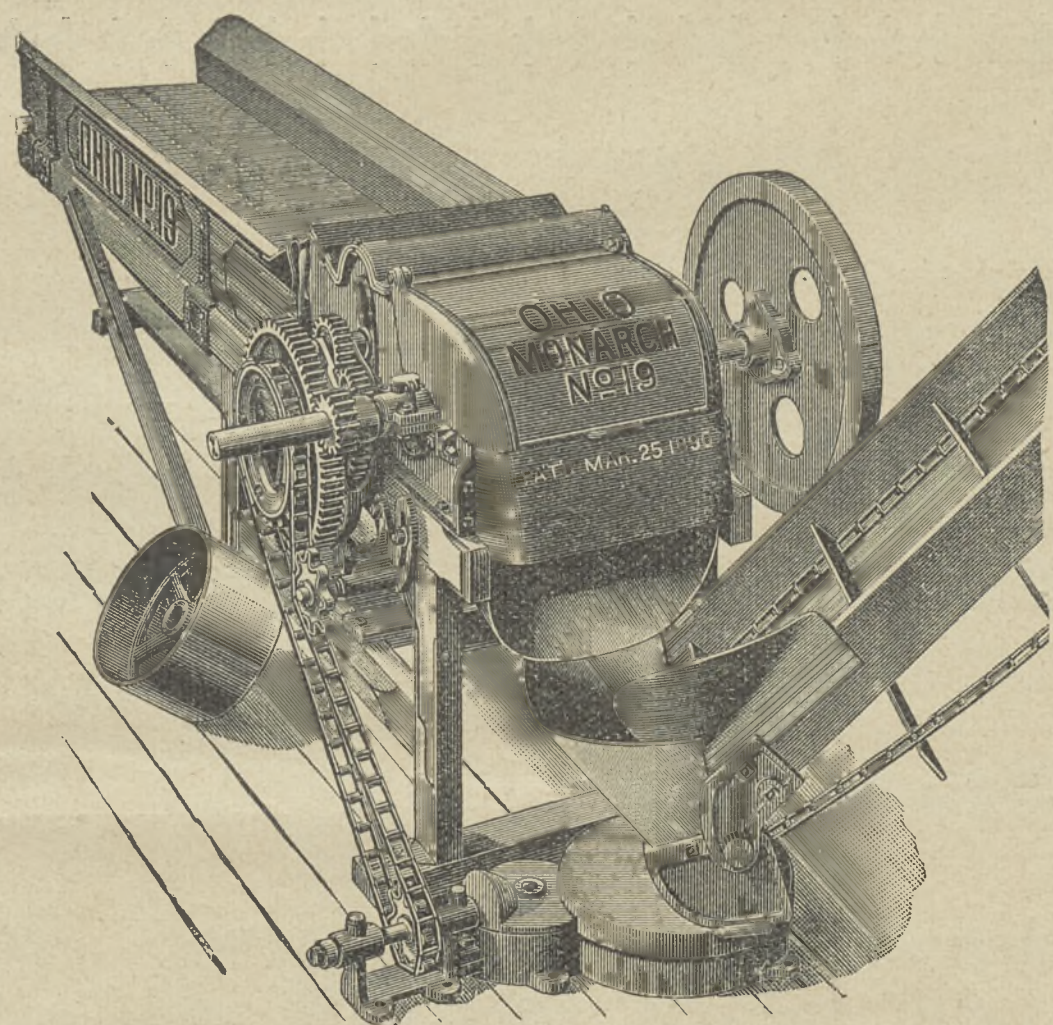
„Ohio“ tengersizártépgép.
