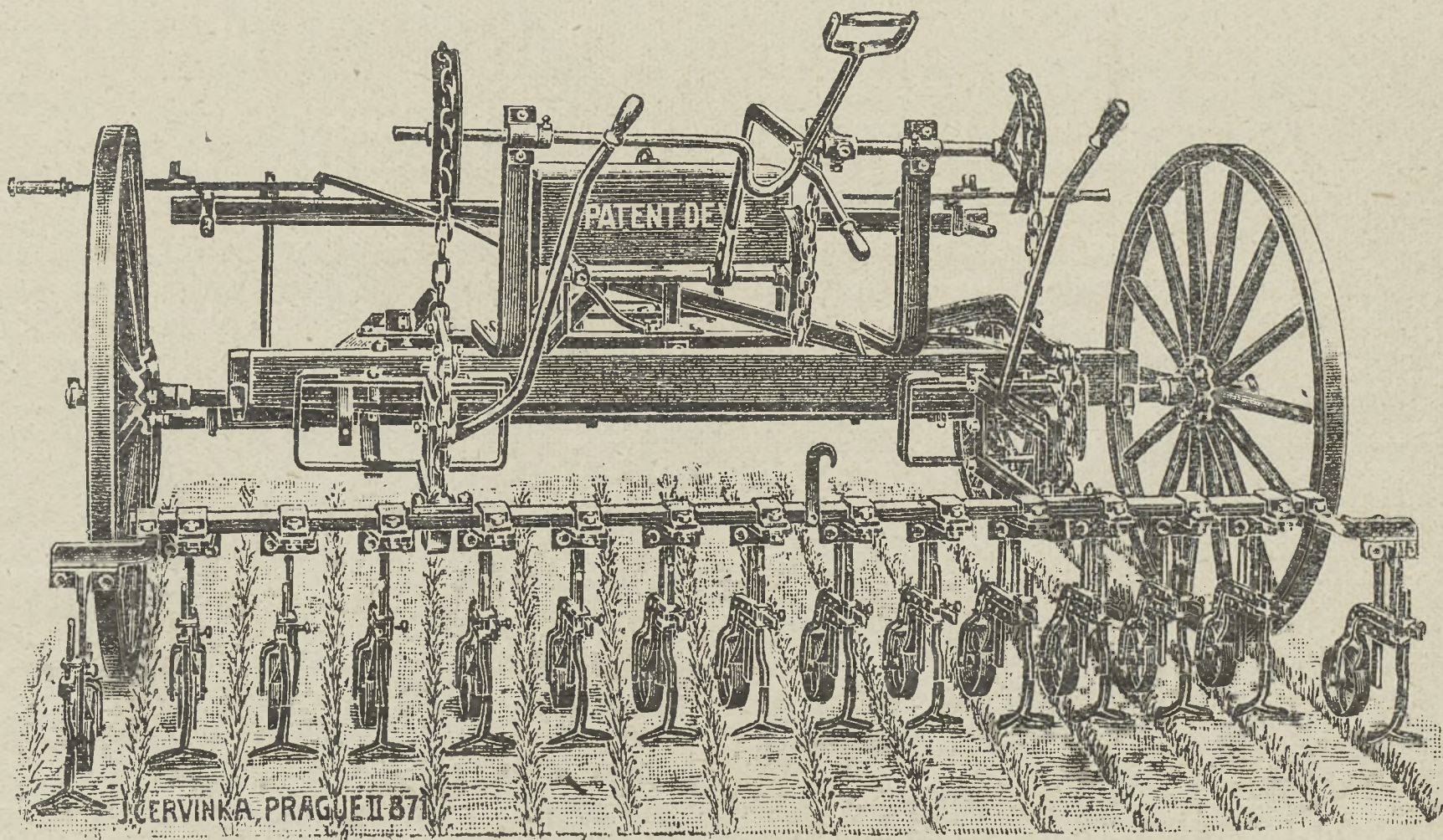
71-ik ábra. Cservinka gabonakapológépe. Deyl szabadalma.
