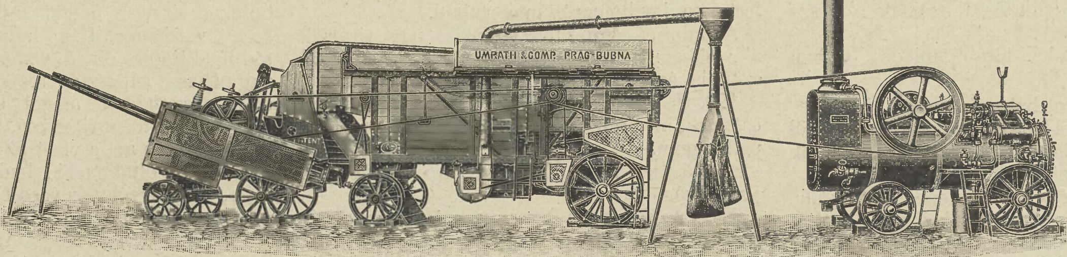
44-ik ábra. Umrath-féle gőzcséplőkészlet forrógőz lokomobillal.
