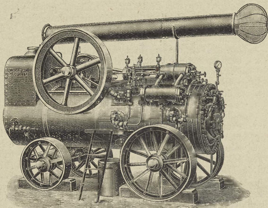
43-ik ábra. Umrath-féle szállítható forrógőzlokomobil kihuzható csöveskazánnal.
