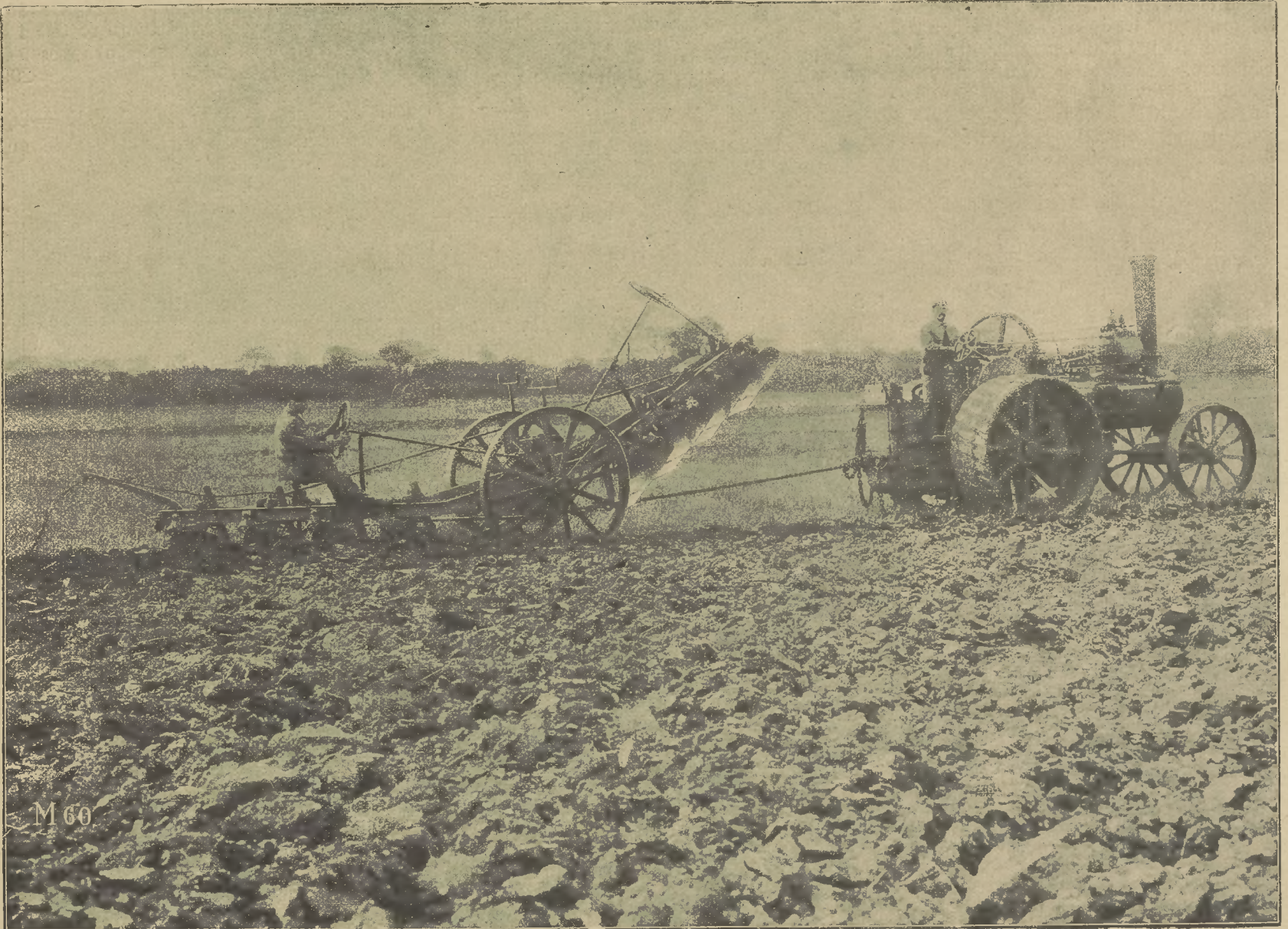
37-ik ábra. Fowler magánjáró gőzekéje.
