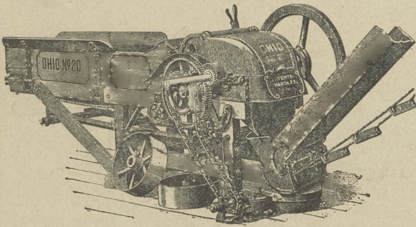
„Ohio“ eredeti amerikai tengeriszártépőgép egszersmind zöldtakarmányapritó- és szecsázó-gép.
