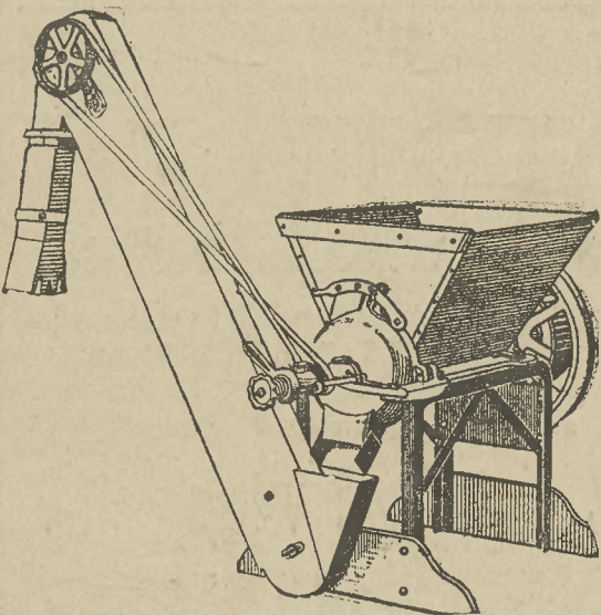
„Ohio“ eredeti amerikai tengeriszártépőgép egszersmind zöldtakarmányapritó- és szecsázó-gép.
