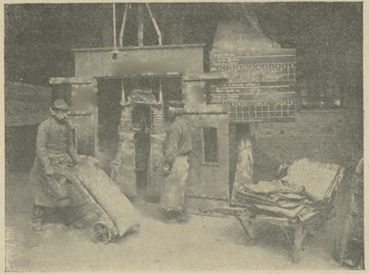
17-ik ábra. Thomassalak-örölő malom.
