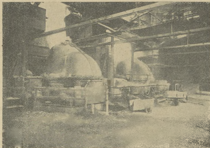
13-ik ábra. A Thomassalak előállításá vasolvastásnál.
