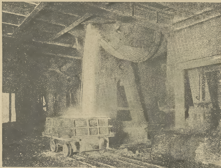
14-ik ábra. A Thomassalak kiömlése kocsikba.
