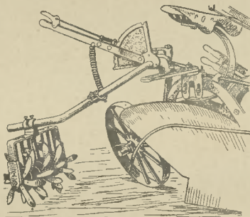
40-ik ábra, Kramer boronával egyesített amerikai ekeje.
