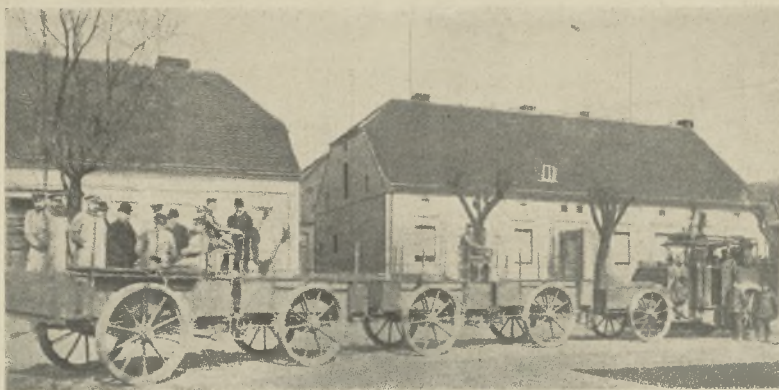
21-ső ábra. Sínpar nélküli haladó országúti vonat. A seeföldi Frohbalgesellschaft gyártmányá.
