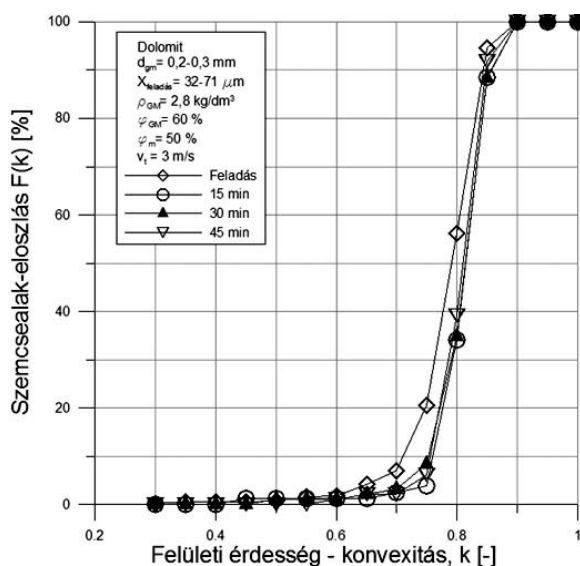
4. ábra: A konvexitás szerinti alakeloszlás változása a tartózkodási idővel, SI=3,94 \cdot 10^{-7} Nm esetén
