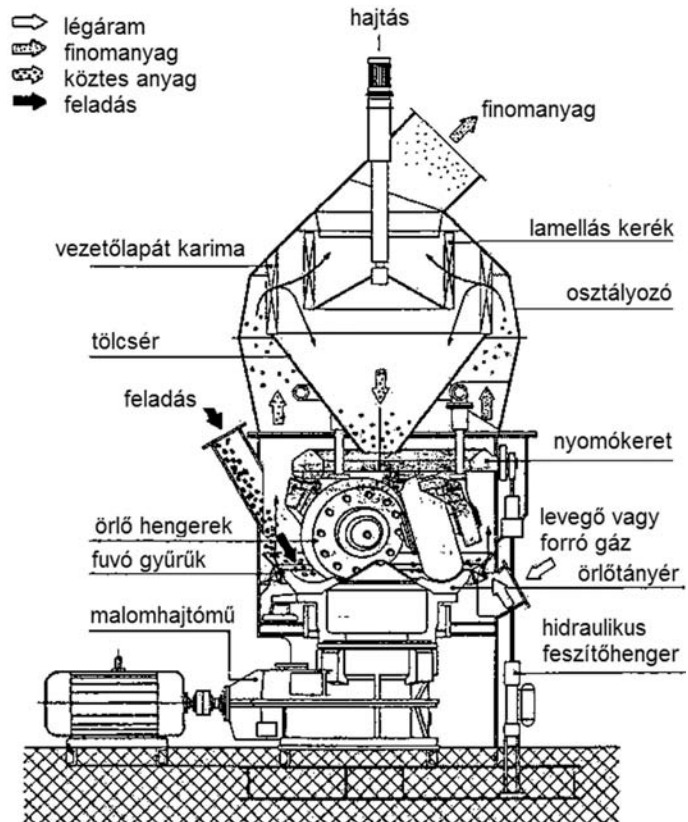
1. ábra: A gyűrűs malom szerkezeti felépítése
