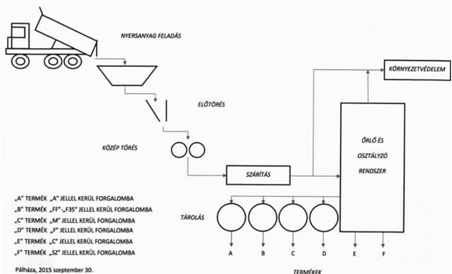
1. ábra: Pálházi perlit-előkészítési technológia
