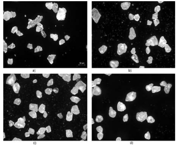
7. ábra: Mikroszkópi felvételek a feladás (32-71 \mu\text{m} ) és alakformált szemcsékről, SI=9,35 \cdot 10^{-6} Nm mellett a – feladás, b – 4 min, c – 8 min, d – 12 min
