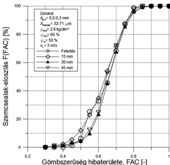
1. ábra: A gömbszerűség hibaterülete szerinti alakeloszlás változása a tartózkodási idővel, SI=3,94 \cdot 10^{-7} Nm esetén
