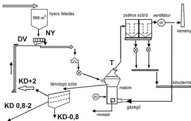
2. ábra: A mézskő előkészítőmű vizsgált technológiája
