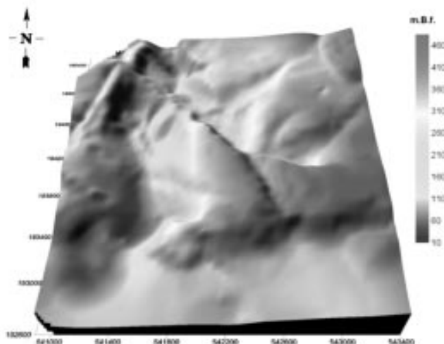
2. ábra: Az Úrkúti Mangánérc Formáció fekkijének domborzatmodellje
