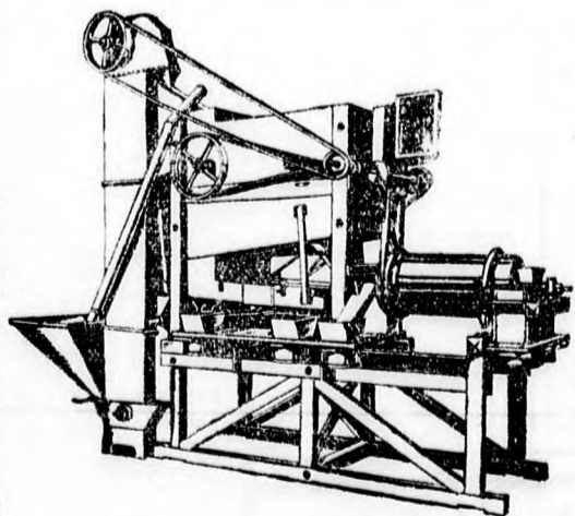
Kombinált „NOVA” vetőmagtisztítógép
