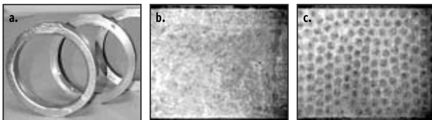
6. ábra. Öntéssel készült erőmérőgyűrűk keresztmetszete: erősítés nélküli (a), közvetlen szálerősítéses (b), duplakompozit (c). A gyűrűk belső átmérője 3 inch, vagyis 76,2 mm.
