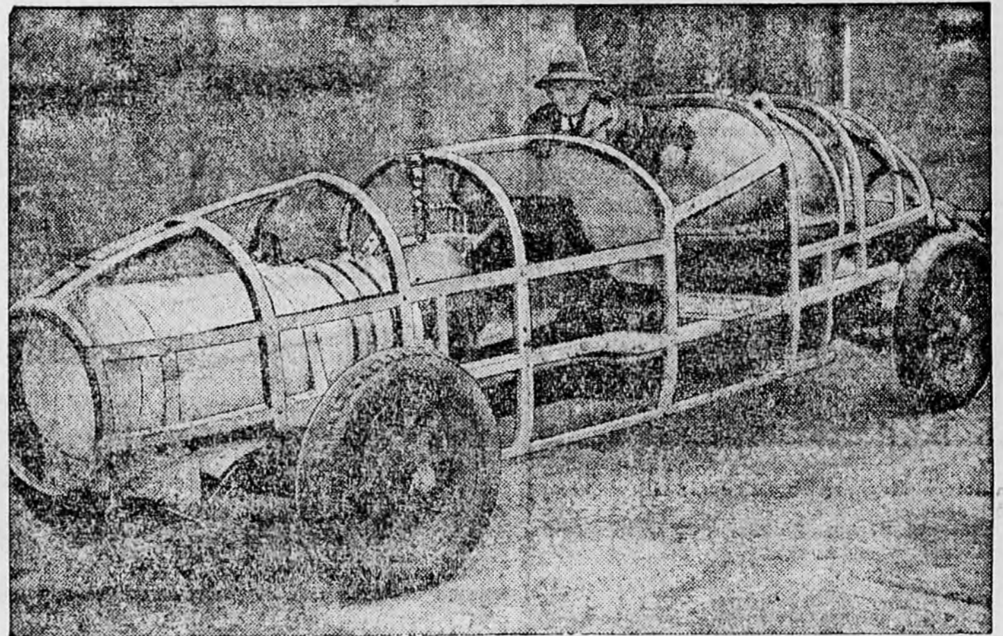
Heyland dr. kiváló német technikus által készített új rakéta-autót most mutatták be a szak-köröknek Berlin-Britzben. Az új csodagépet a nagyközönségnek májusban mutatják be a Berlin-Tempelhofi repülőtéren.
