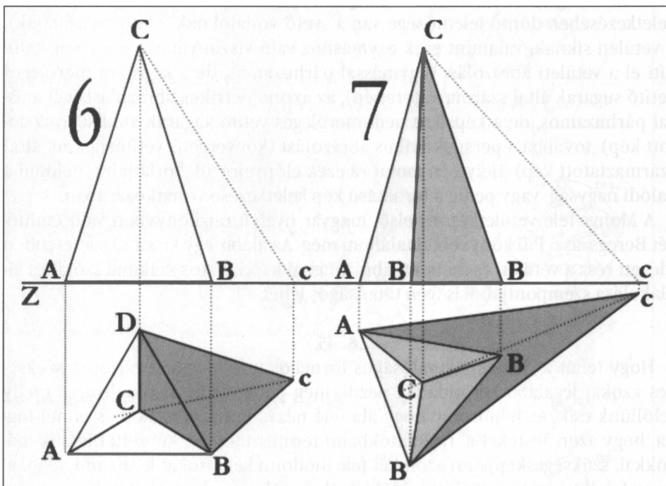
4. ábra. A Monge-féle vetületek keletkezése
