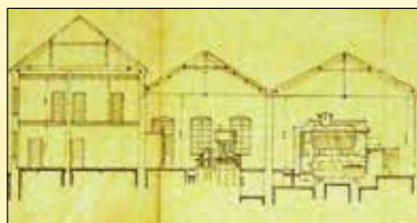
A villanytelep rajza 1934-ből – Molnár Tibor építész képeiből
