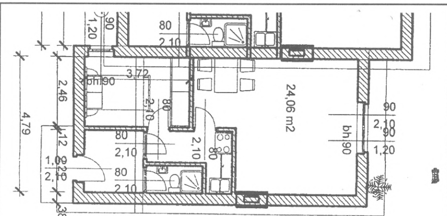
Egy közel 50 m 2 -eres összkomfortos szociális lakás előzetes tervrajza. 4-5 ilyen vagy ehhez hasonló lakás épülhet meg ebben az évben a Bányató utcában.
