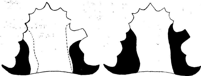
3. ábra \bar{e}(p) ; ----- : a (v)\bar{i}(v) határa.
