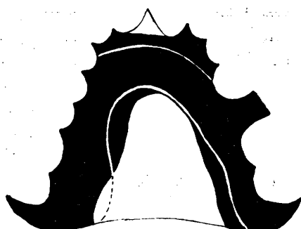
8. ábra ( b\bar{a} ) n(\acute{a}) ; a fehér és szaggatott vonal az n határa.
