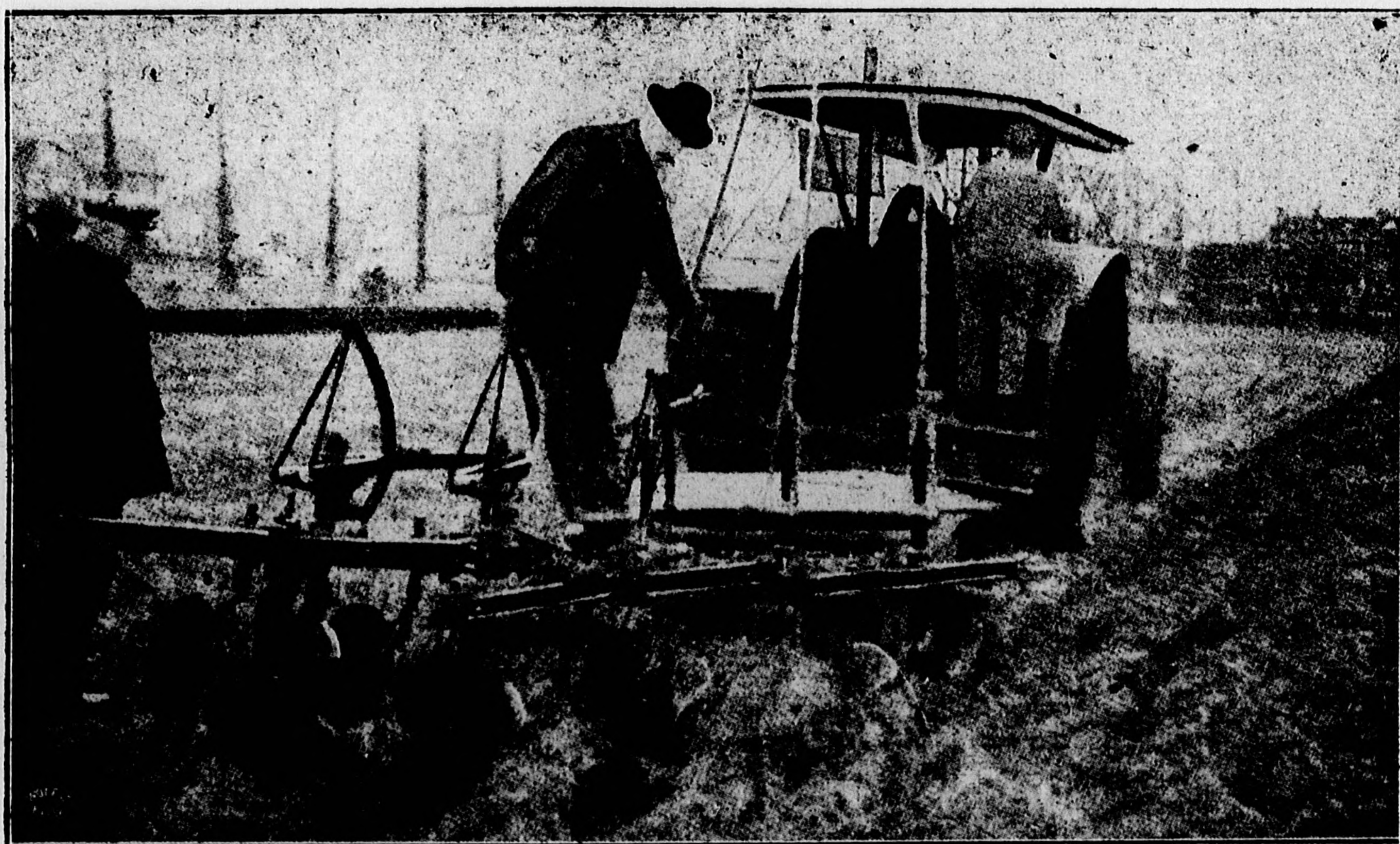
Amerikai 25 lóerejű motoros eke, amely 72 perc alatt felszánt egy hektár szántóföldet.
