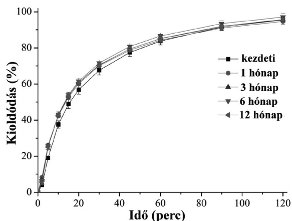
3. ábra: Szálképzett ASD-t tartalmazó, körforgós tablettázógéppel gyártott tabletták kioldódás profilja és hosszú távú stabilitás tesztje. Paraméterek: 900 ml 0,1N HCl, 37 \pm 0,5^\circ\text{C} , USP II lapát, 100 mg dózis, 50 rpm forgási sebesség.
