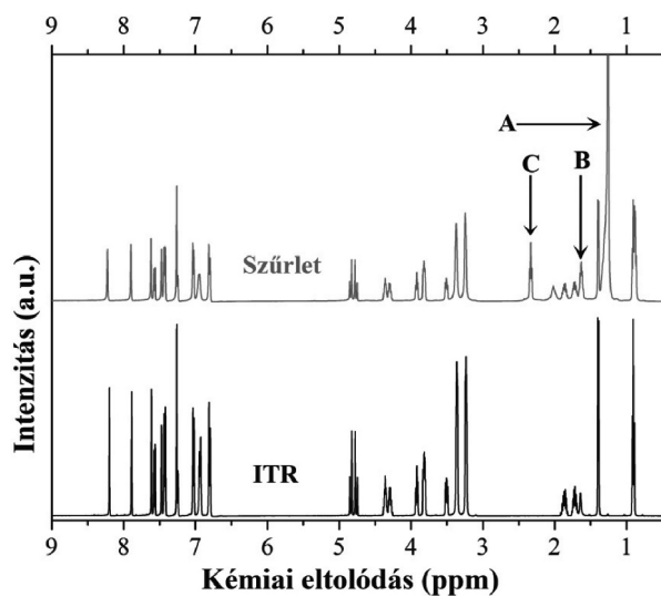
8. ábra: ITR és a szűrlet nukleáris magrezonancia spektroszkópiás spektruma (500 MHz, CDCl 3 ). A, B és C jelöli a „sztearát-lánchoz” tartozó csúcsokat.
