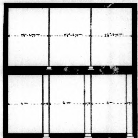
II. ALAPRAJZ
