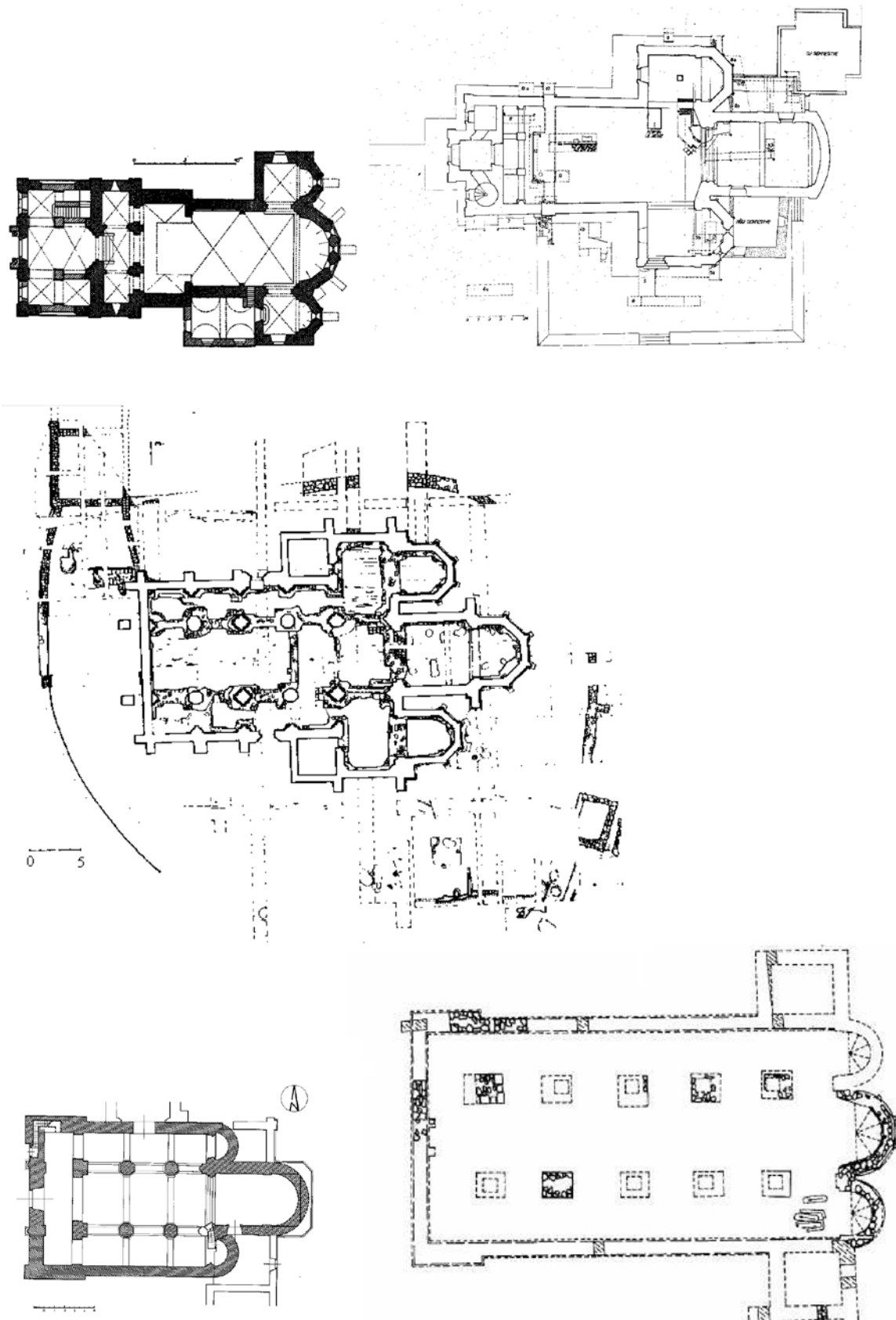
1. ábra. Premontreai prépostságok megkutatott alaprajzai I.: Bény, Jánoshida, Ócsa, Túrje, Majk
