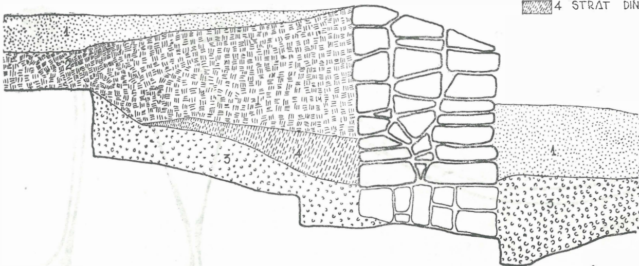
Fig. 4. — Secțiunea peretelui nordic al șanțului I al cetății dacice din Valea Casinului.
