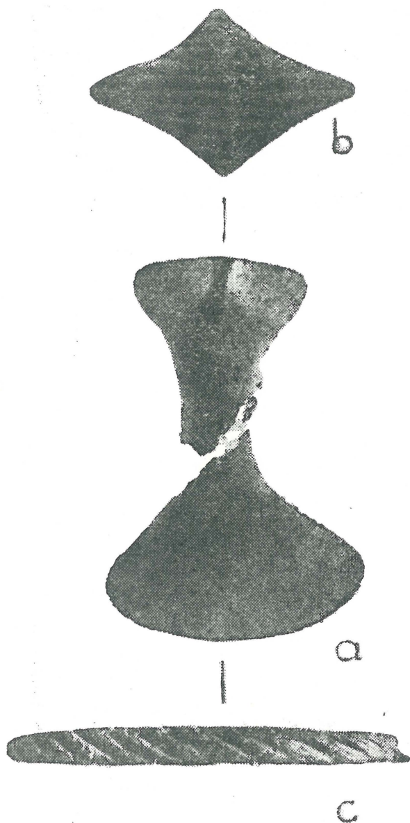
Fig. 1. Instrument de lut ars pentru ornamentarea ceramicii, descoperit la Cozia. In ansamblu (a), terminația romboidală a minerului (b), marginea arcuită crestată a instrumentului (c). (a = 1,14, b = 1,65, c = 1,57 mărimea naturală).
