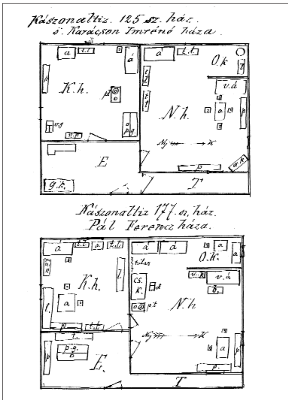
4-5. ábra ROEDIGER Lajos 1913. évi kászonaltízi felmérései a Székely Nemzeti Múzeumnak. E - ereszt; Ka - kamra; K.h. - küs ház; N.h. - nagy ház; O.k. - oldalkamra; T - tornác; a - asztal; á - ágy; b - bölcső; g.k. - gabonakar (szuszék); l - láda; p - fakanapé (pad); p.g. - pincegrádics; p.t. - platten (takaréktűzhely); s - szék; t.l. - tulipános láda; ü.k. - üvegkasztén; v.á. - vetett ágy; v.g. - varrógép.
