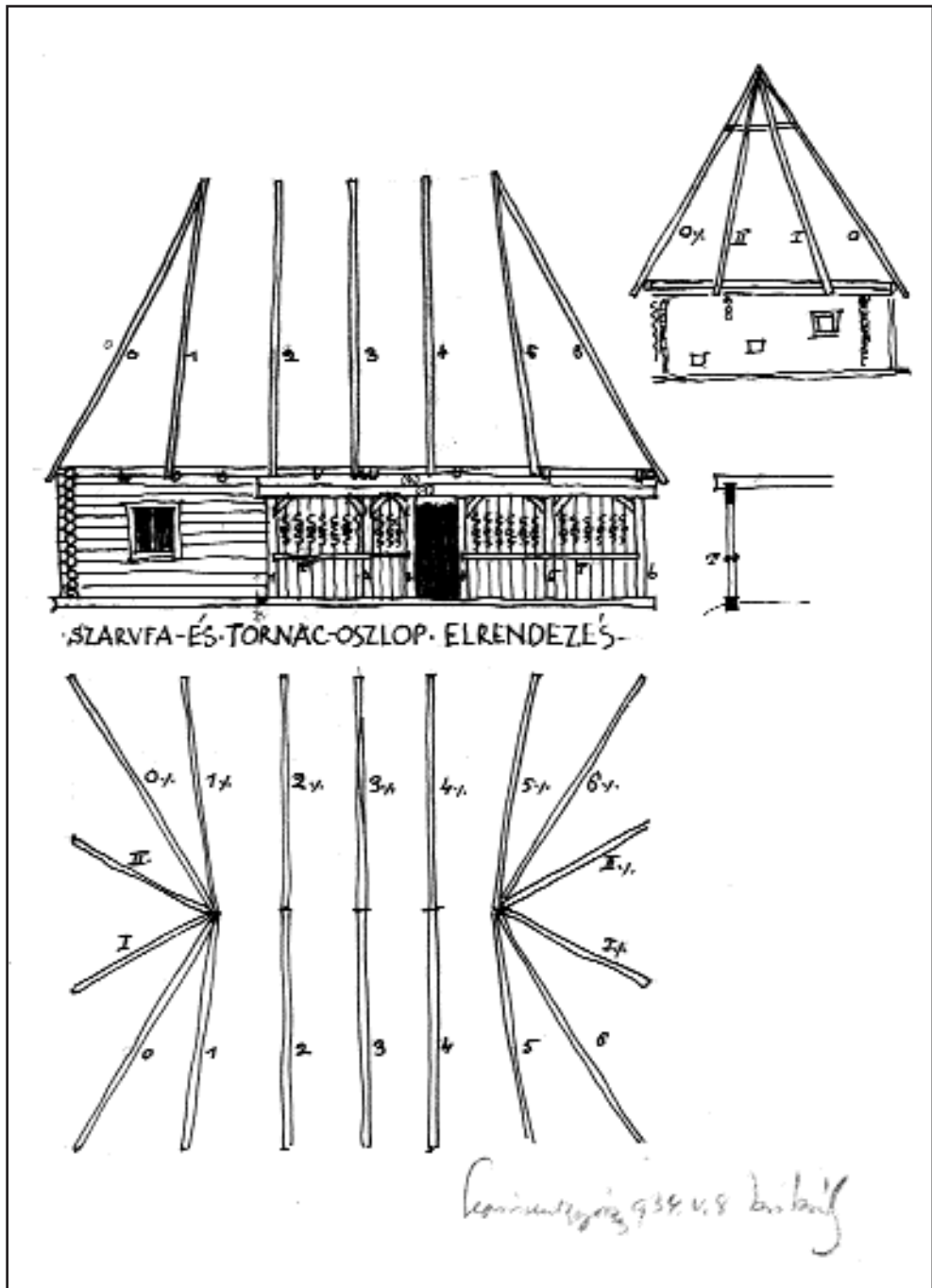
14. ábra A Csíki ház szarufáinak és tornácoszlopainak elrendezése (KÓS Károly Sepsiszentgyörgyön befejezett rajza, tussal utánhúzva).
