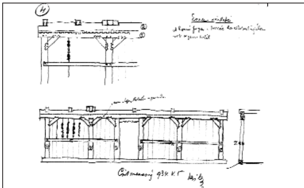
15. ábra Részletrajz a Csiki ház ereszeről (KÓS Károly csikmenaszói felvétele).
