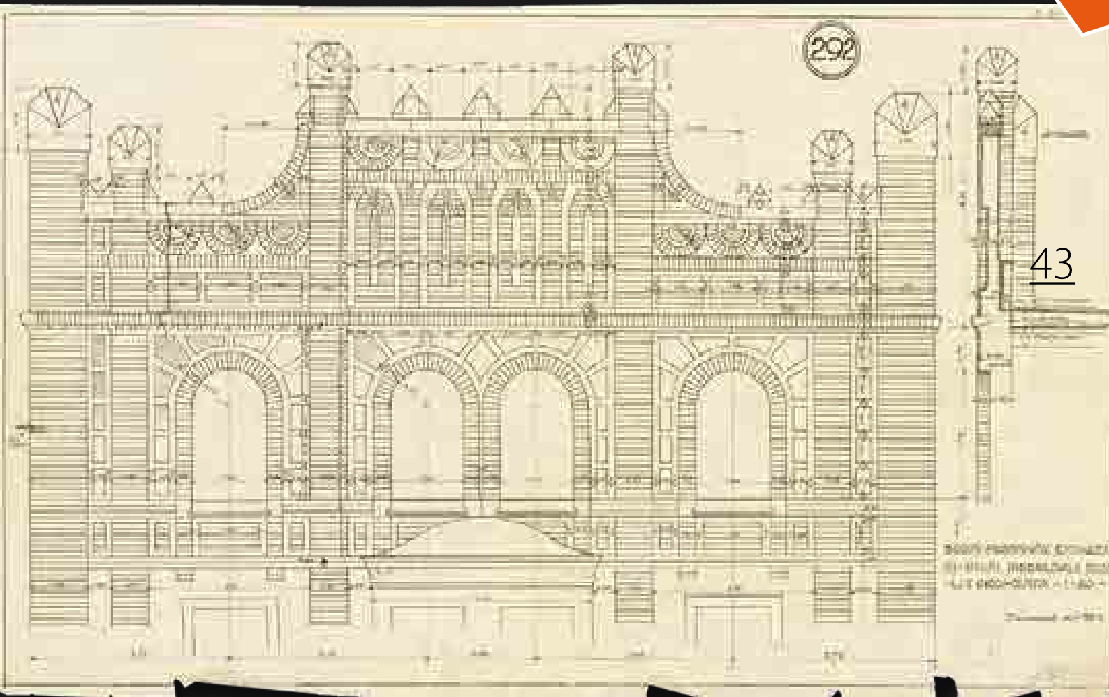
Eredeti tervrajz az épületről (1924–1925)
