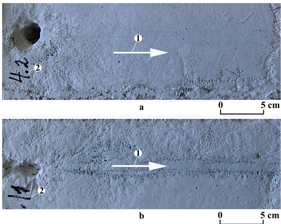
7. kép: A gipsztáblák oldódása, ha a vízáradás oldalról a fekére (4/1 jelű gipsztábla) és, ha a vízáradás fentről a fedőre oldalról (4/2 jelű gipsztábla) történik
