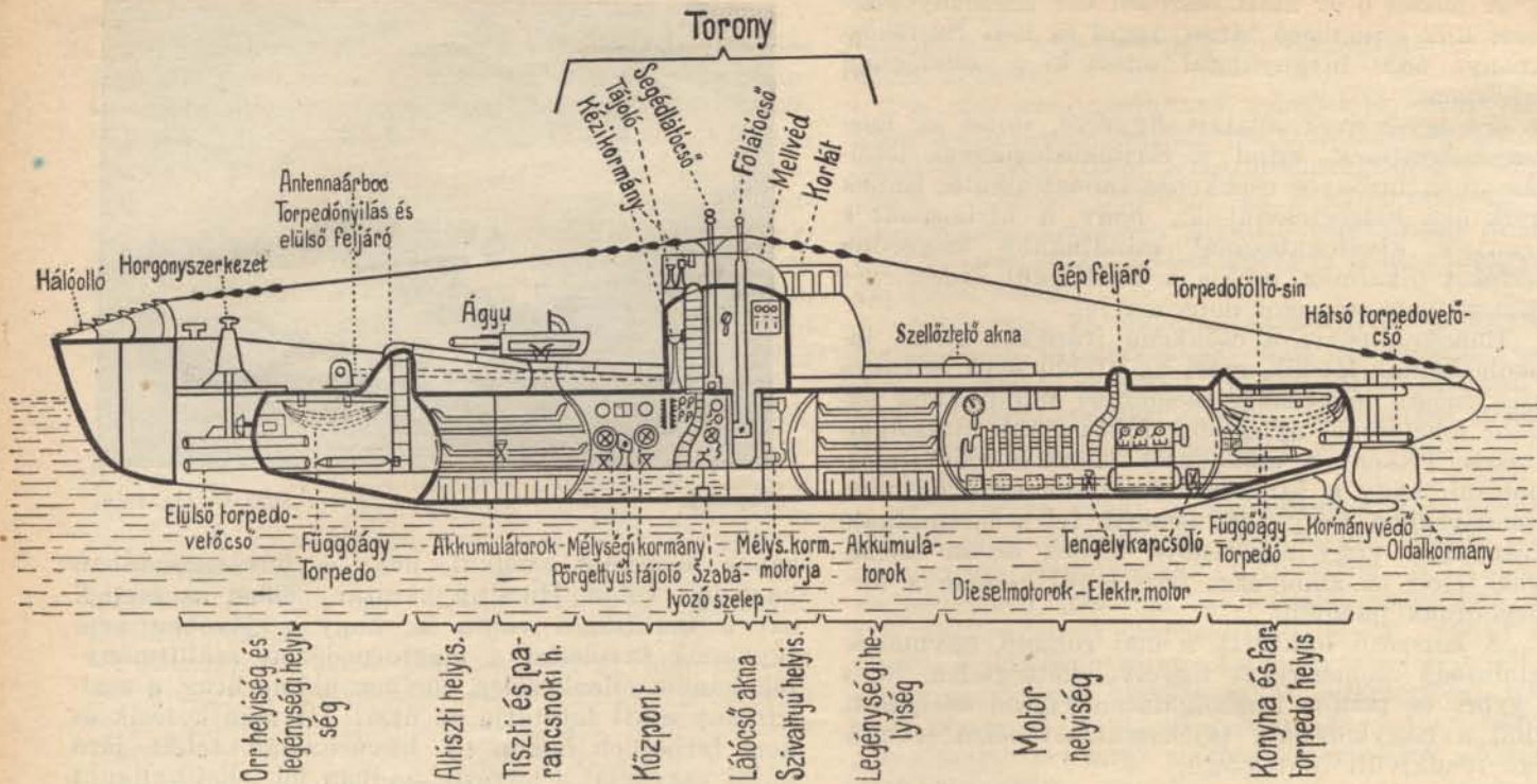
Búvárnaszád keresztmetszete.
