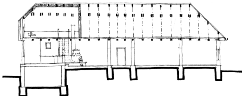
Itt és a szemközti oldalon: Backamadaras saját családi ház; homlokzat, alaprajz, metszet, vázlatok, valamint az épülő és a kész ház részletei
