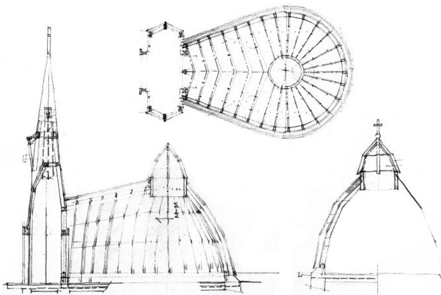
Tolvajostető (Románia), kápolna alaprajza és metszetei (vázlattev.)
