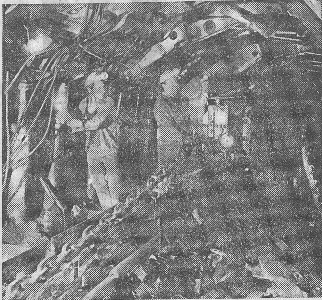
Frontfejtés a várpalotai bányáüzemben
