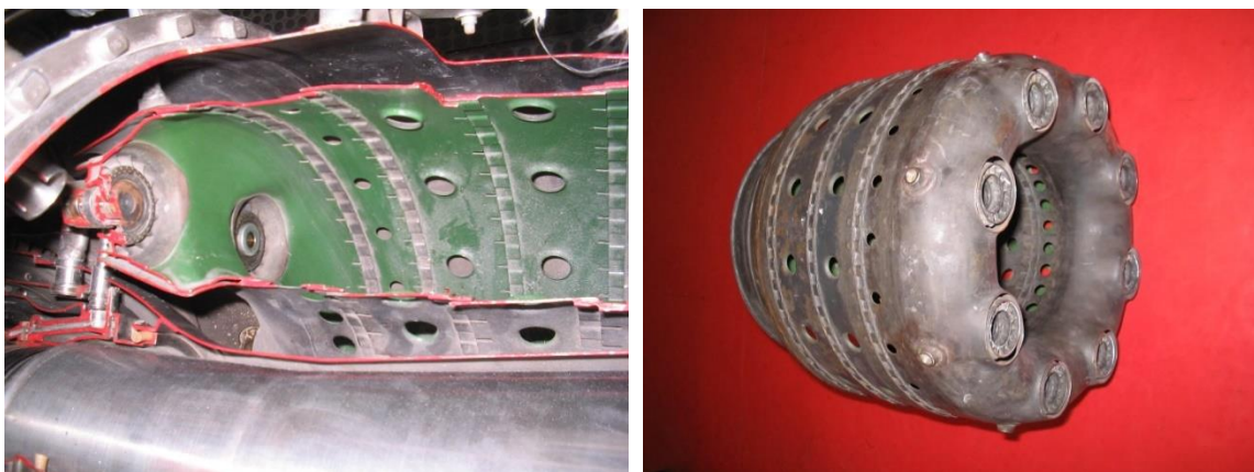
4. ábra Bal oldalon gyűrűs égőtér, jobb oldalon a tűzcső maga (saját kép)
