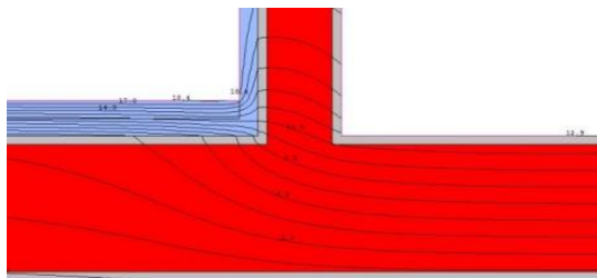
Vízszintes metszet, hőeloszlási görbe. 331. o. Belső oldali hőszigetelés áthúló falszerkezetet eredményez, hőhidasság várható a válaszfal túloldalán.
