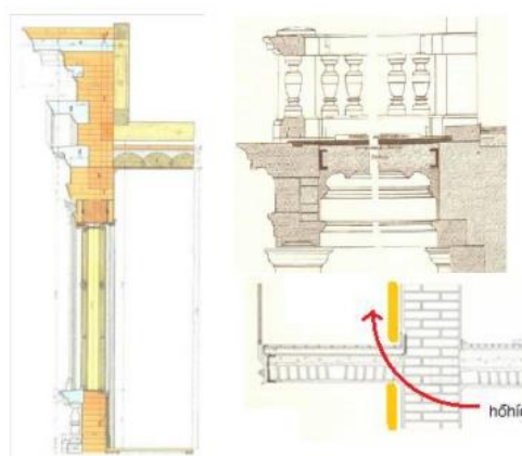
Historizáló épületek homlokzatának ereszkiképzése, Budapest, VII. ker. Szentkirályi u. 22., Metszet: BFL, Legfelső emelet, zárópárkány, erkélyalakítás, függőfolyosó külső oldali hőszigeteléssel; Forrás: Fülöp Zsuzsanna
