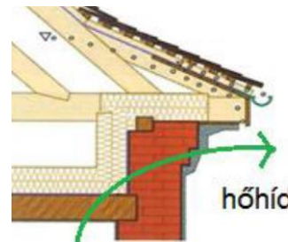
Padlásfödém hőszigetelése után a főpárkány hőhidassá válik, páralecsapódás a csapos-fafödém gerendáinak felfekvésénél.
