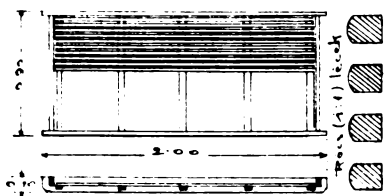
Cserény ránzeti és hosszmetzeti rajza.
