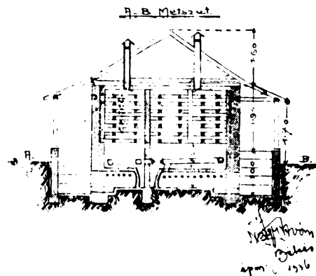
Alaprajzon A—B vonalban átmetszett aszaló a fűtő- és aszaló-terek méreteit türteti fel.
