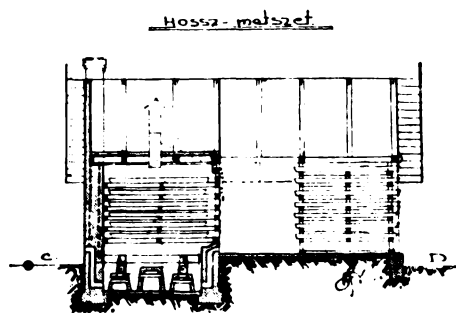
Hosszmetszetben jól láthatók az üzemben levő cserények.
