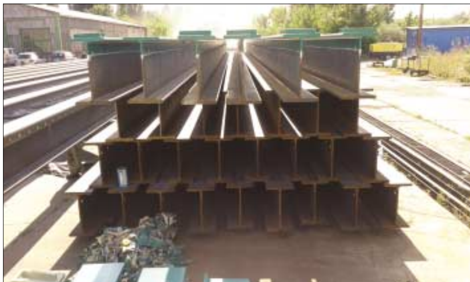
Az Aranyhegyi patak hídjának tartóbetétei kifúrva a készülő korrózióvédő bevonattal
