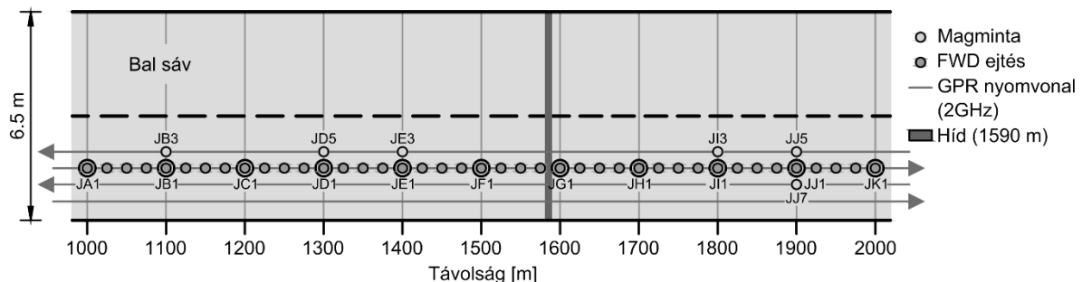
1. ábra: A kísérleti útszakasz méréseinek térbeli elrendezése.
