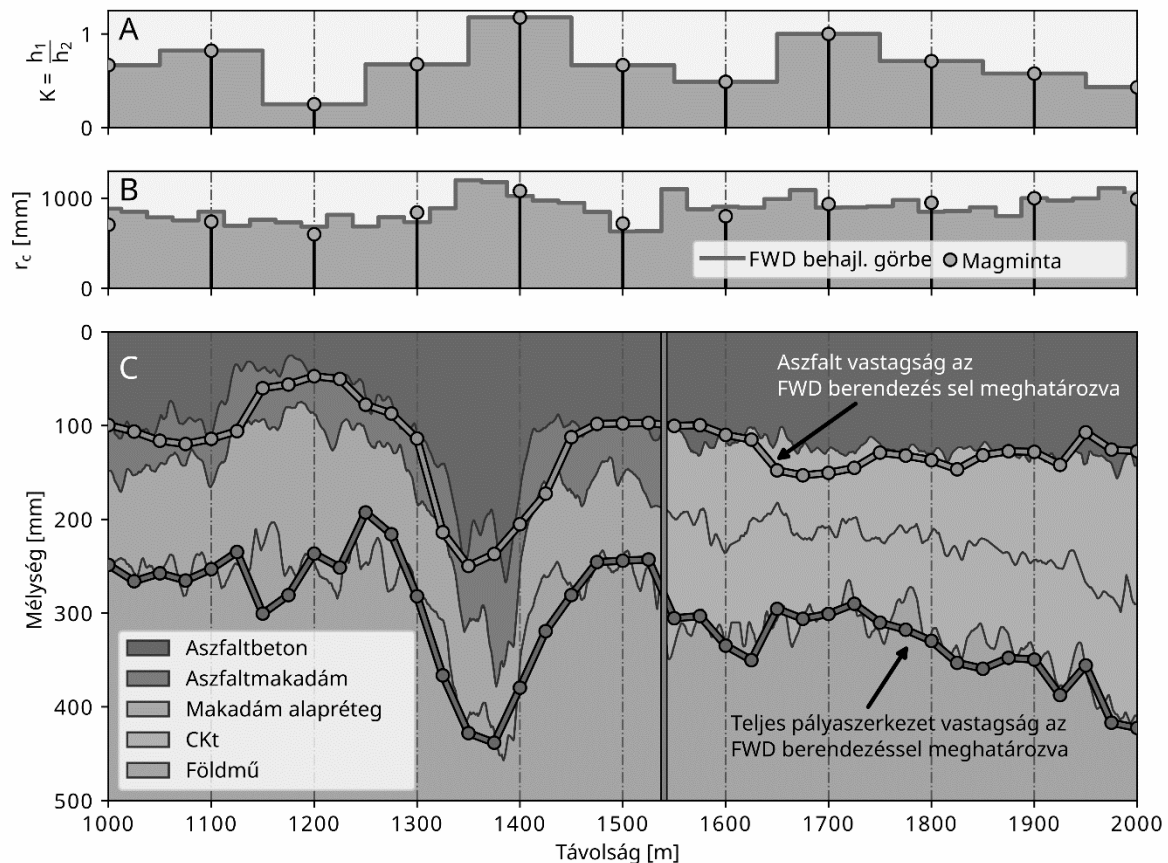
6. ábra: Teljes és aszfaltburkolati rétegvastagság FWD-adatok alapján.
