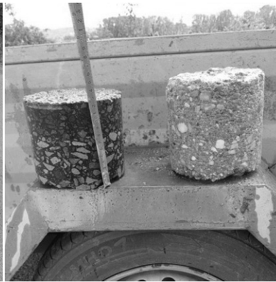
b) aszfalt és Ckt rétegekből származó fúrt minták
