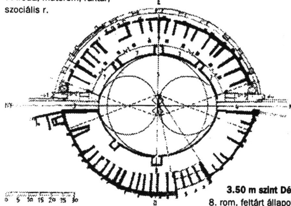
A körszínházi romok feltárt állapota és kőtári alaprajza.
