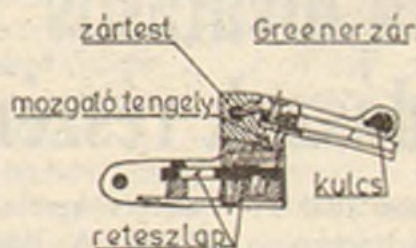
3. sz. ábra. Greener-zár
