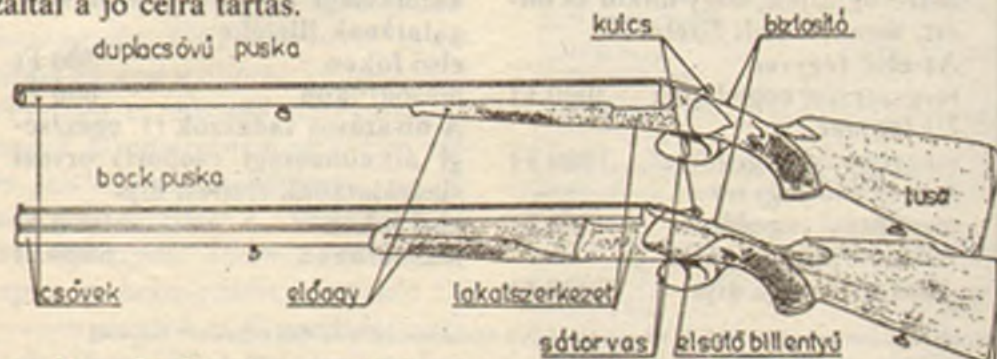
5. sz. ábra. Sörétes fegyver fő részei
