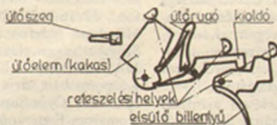
4. sz. ábra. Sörétes fegyver elsütőszerkezeté
