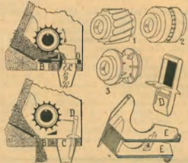
169. ábra. Dehne-féle toléshengernek.
