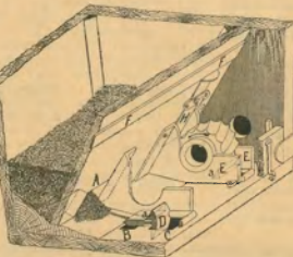
168. ábra. Vetőálda Dehne-féle toléshengerrel.
