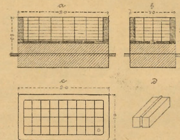
18. abra. Zománczott kőagyatékhoz teljes házak, mosókonyhák stb. számára.
