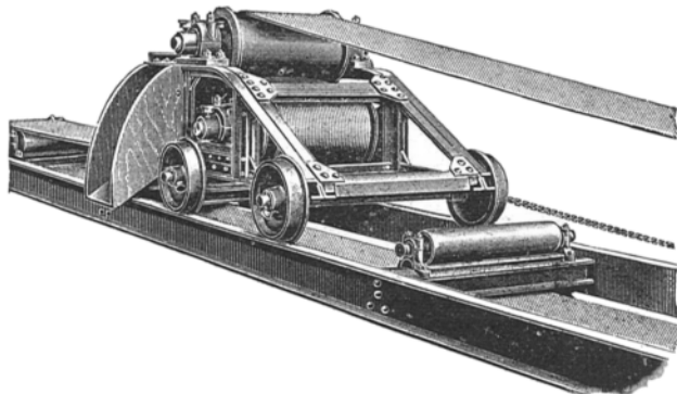
Szalagszállítóberendezés szabadalm. automatikus elosztókocsival
