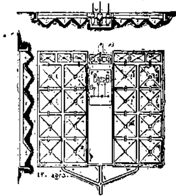
Ülepitő berendezés-berendezés vázlatja.
