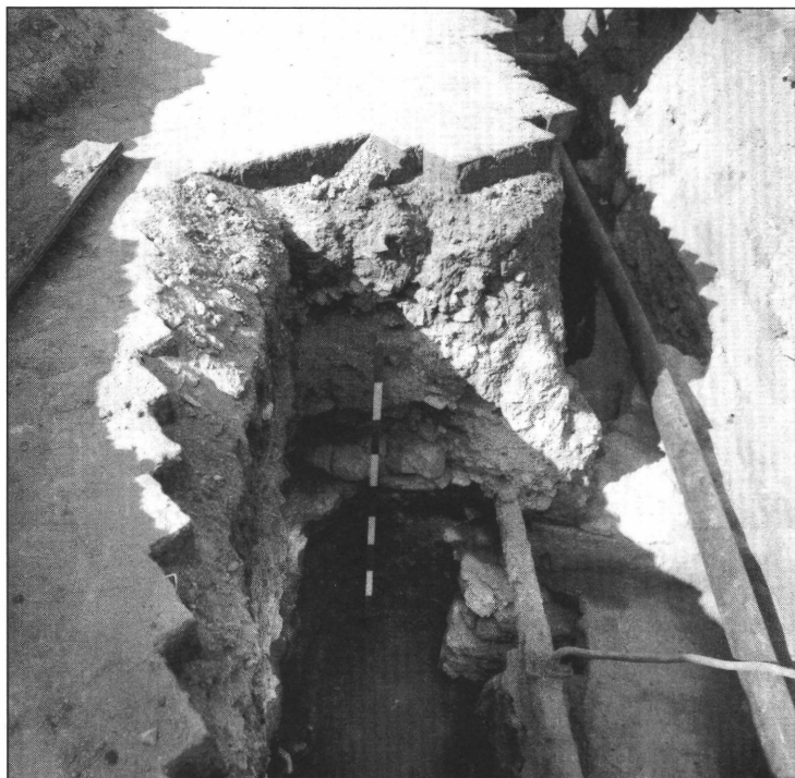
6. kép. Az északi mellékrajó sávalapozásának részlete, mely két-két római pillér között húzódik K-ről. A habarcspadló és kőpadló részletével, melyeket az újkori közművek átvágtak.
