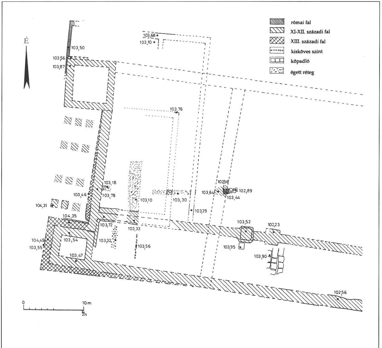
2. kép. A Westwerk alaprajza
