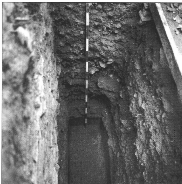
17. kép. A háromhajós templom déli mellékhajójának kibontott alapozásának, ill. utolsó kősorának részlete É-ről
