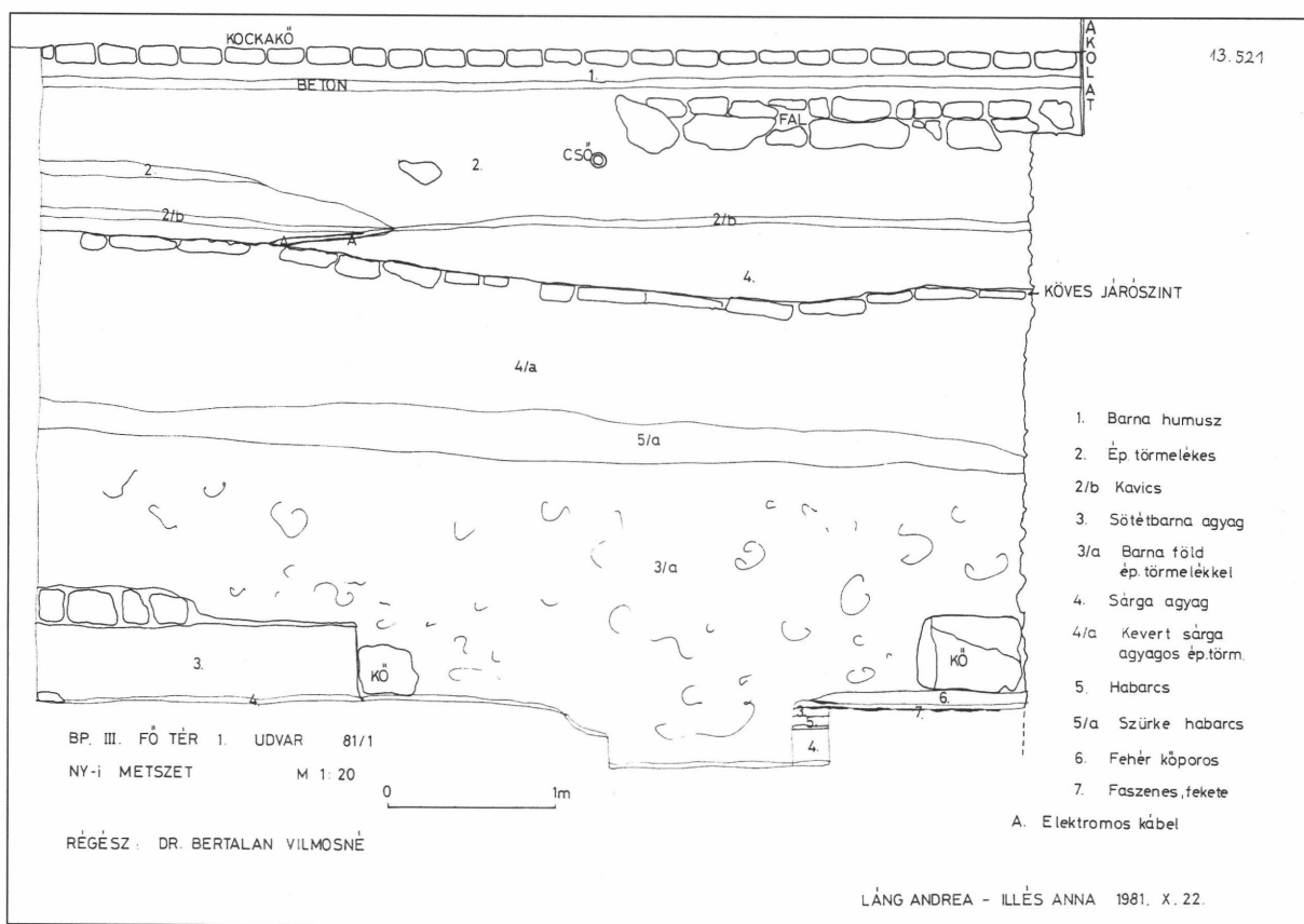
15. kép. A 81/1-es kutatóárok nyugati metszete az altemplom és a kelet-nyugati római fal kibontott részletével, valamint az altemplom kőpadlójának maradványa (6-os réteg)
