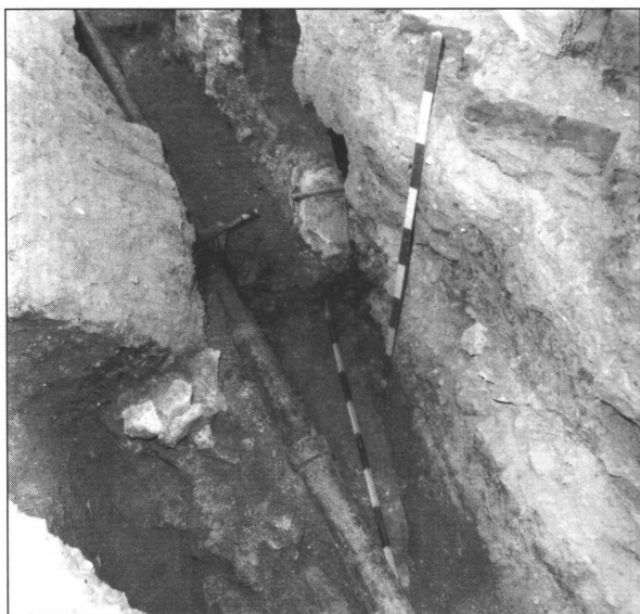
23. kép. A déli torony átépítésekor készült falvastagítás részlete. Az északnyugati sarok és az oszlop alapozása.
