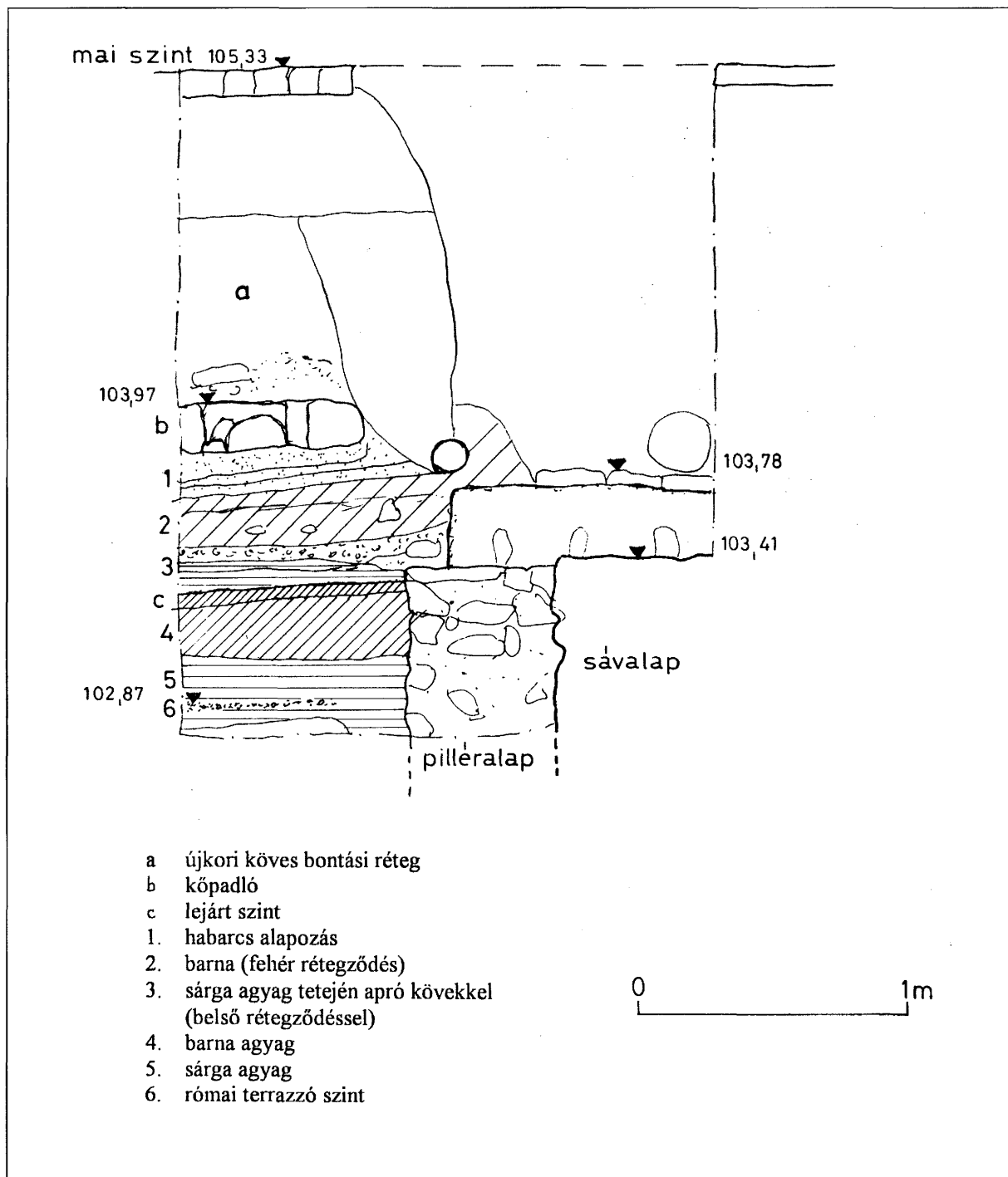
5. kép. Az északi mellékhajó sávalapozásának és pillérének részlete a K-Ny-i közműűárokban és D-i rábontásban. A rábontás és árok nyugati falának metszetrajza.
