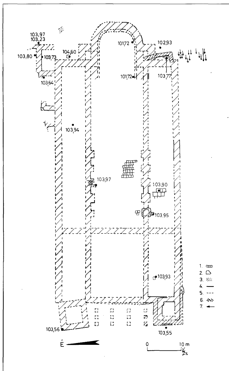
1. kép. A Péter templom kiszerkesztett alaprajza (elvi rekonstrukció). 1. kőpadló, 2. vörös márvány padló, 3. padló alatti habarcsalapozás, 4. feltárt falak, 5. összeköthető falak, 6. árkádív alapozás, 7. sírok (temető)
