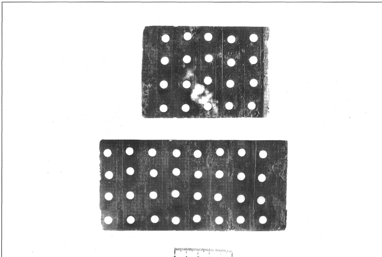
3. kép. A szélszekrény fedlapja
