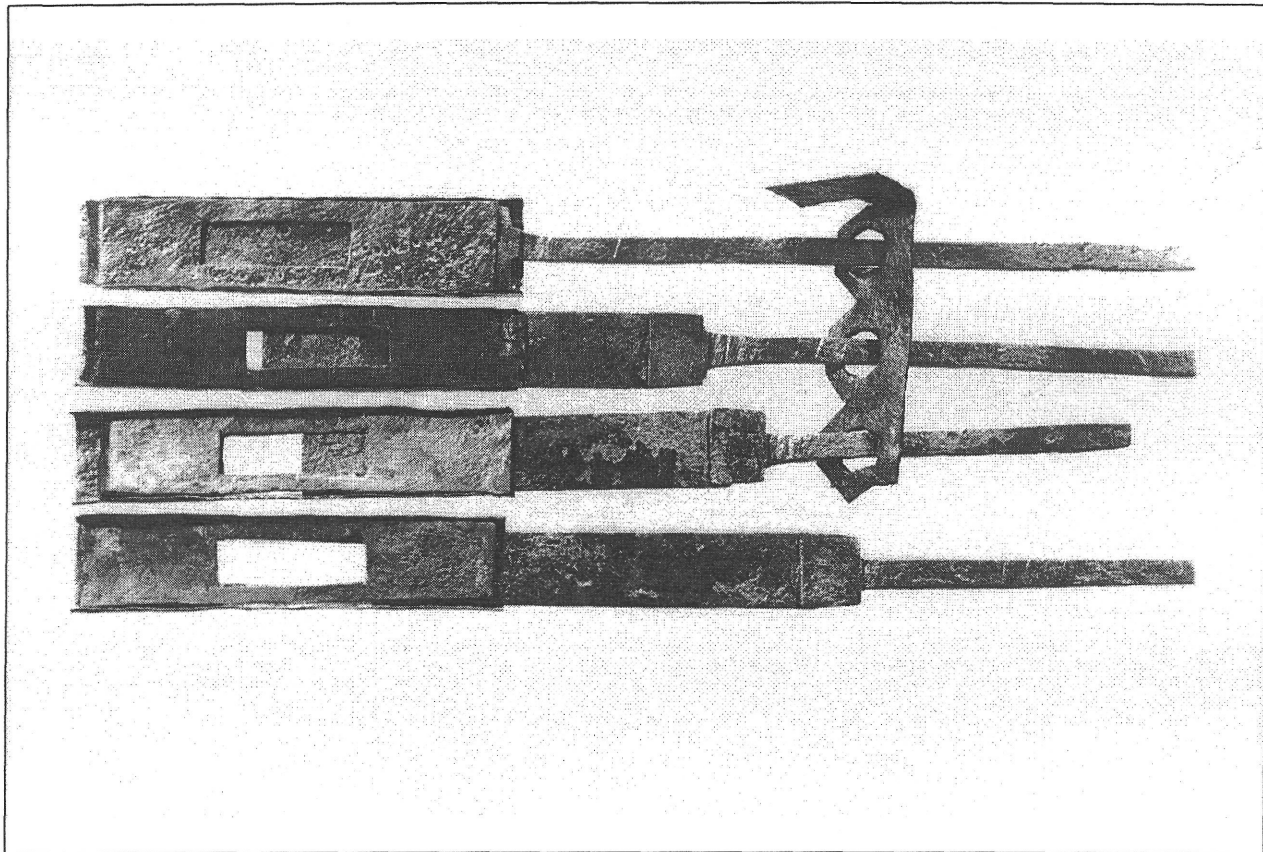
4. kép. Regiszter csúszkák
