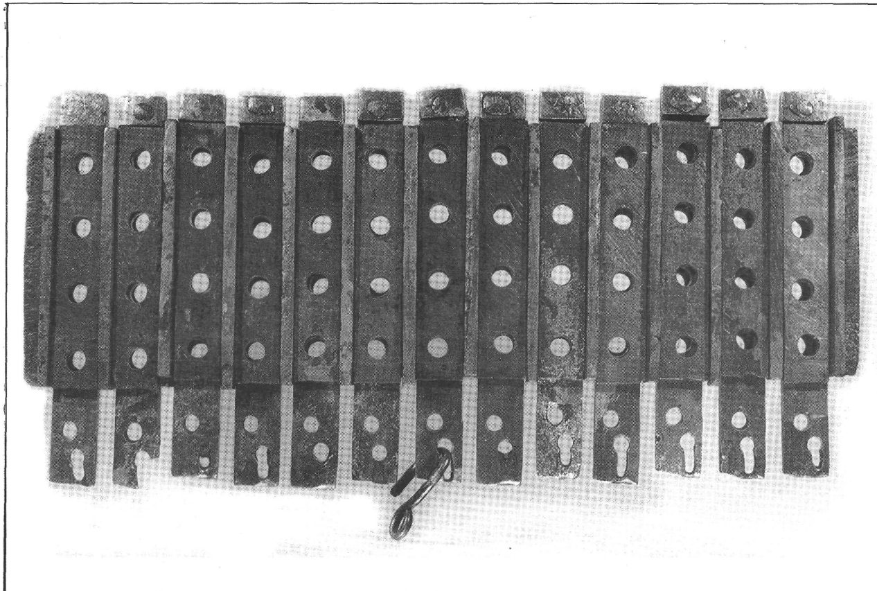
5. kép. Billentyű csúszkák
